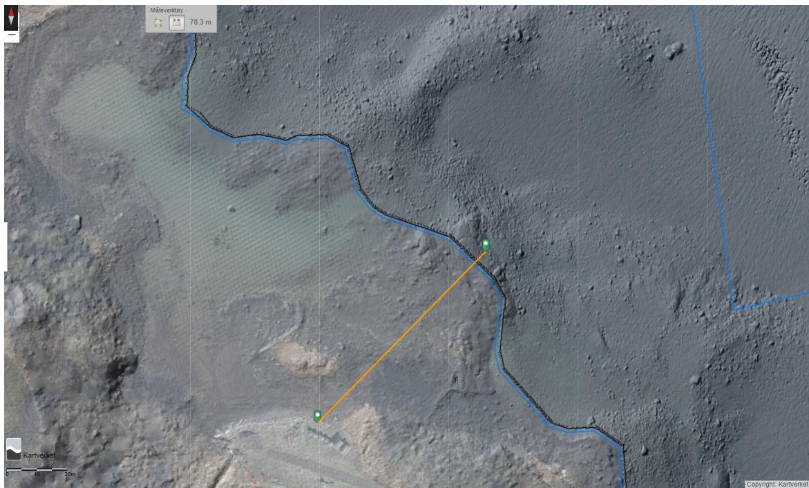
Figur 10 Bathymetri som viser kombinasjon av fjell og morenemateriale som ligger i den langgrunne strandsonen. Avstand fra marbakken til flomålet er rundt 80 meter.
