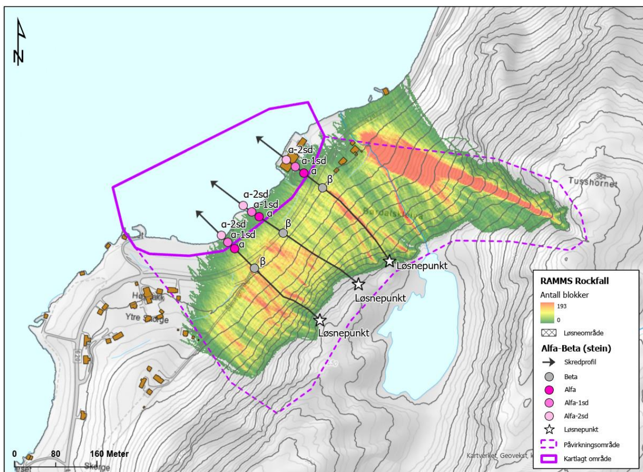
Figur 20. Resultater fra modellering av steinsprangutløp, dynamisk modell RAMMS rockfall (antall steinsprangblokker som passerer hver celle i simuleringen) og empirisk/statistisk analyse (alfa-beta). Utstrekning av kartleggingsområdet kan avvike noe i figuren, se figur 1 og 21 for nøyaktig utstrekning.
