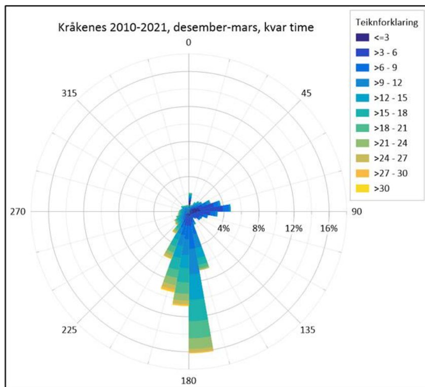
Figur 11. Vindrose for vintermånedene desember til mars.
