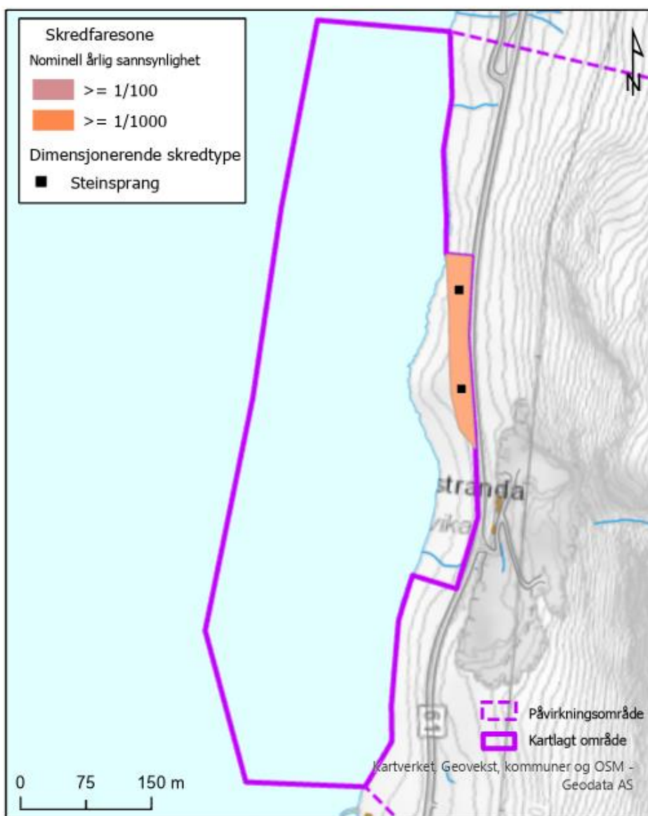
Figur 20. Faresonekart for det kartlagte området. Hele området er vurdert til å ha lavere nominell årlig sannsynlighet for skred enn 1/100 . En del av området er vurdert å ha høyere sannsynlighet enn 1/1000 , og det er knyttet en faresone til dette området.
