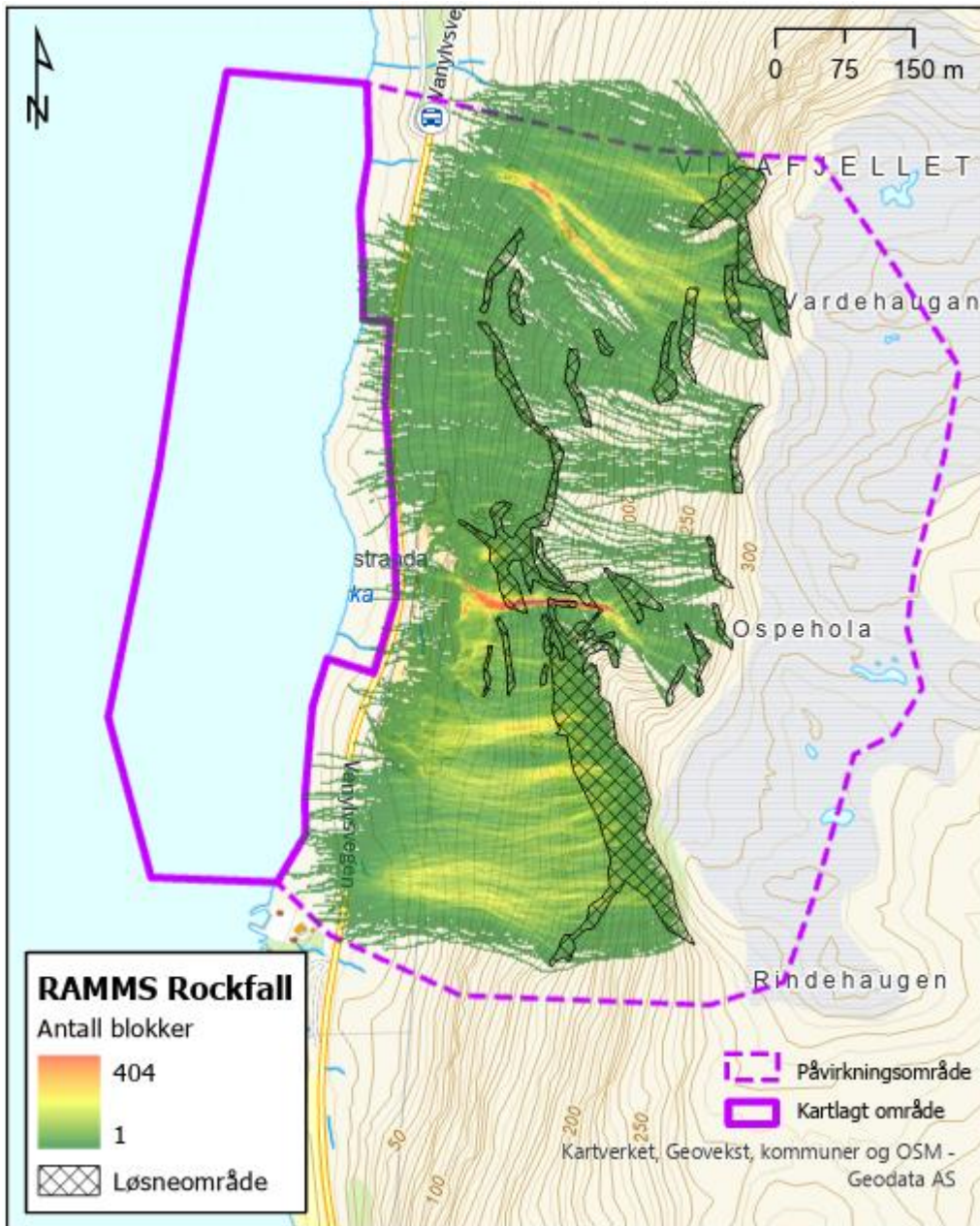
Figur 19. Resultater fra modellering av steinsprangutløp, dynamisk modell RAMMS rockfall (antall steinsprangblokker som passerer hver celle i simuleringen).
