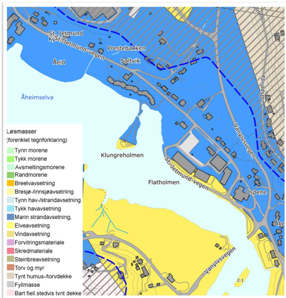
Figur 2: NGUs løsmassekart [2].
